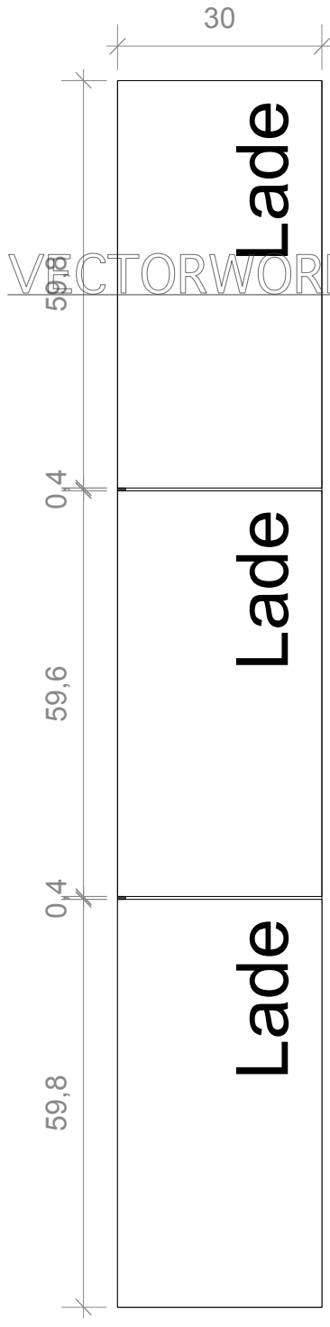
Voorraanzicht Badkamerkast
