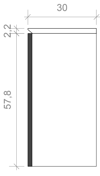
Zijaanzicht Badkamerkast
