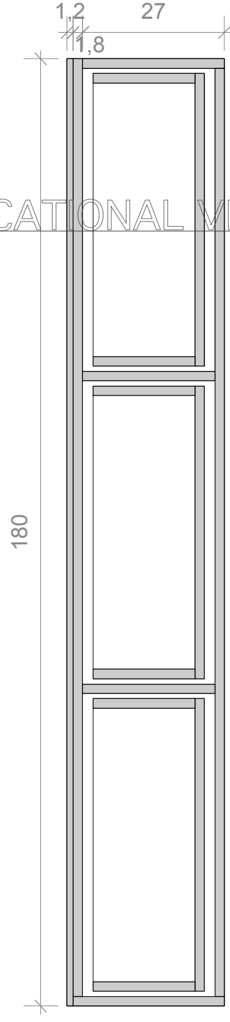
Voorraanzicht Badkamerkast
