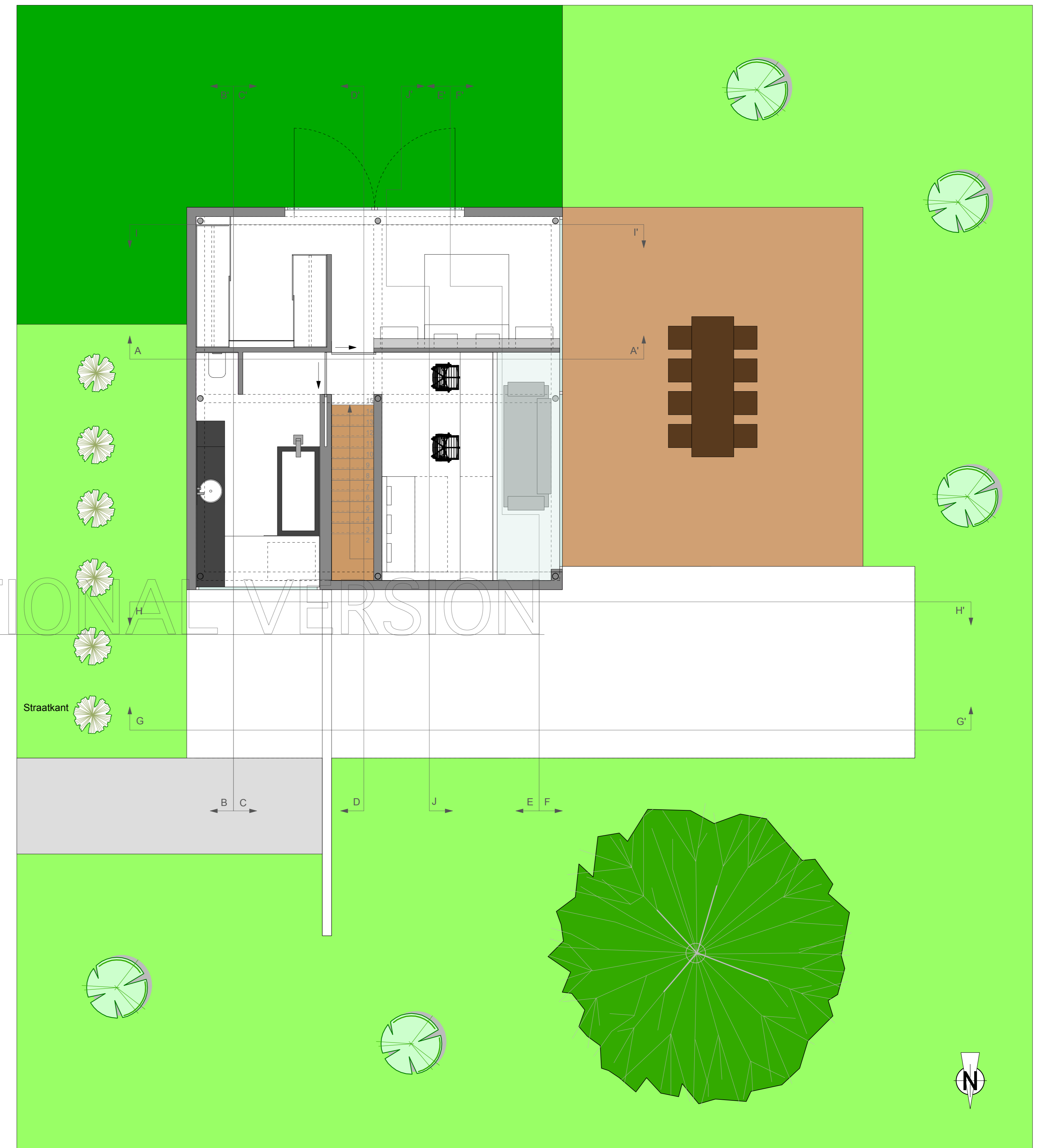
Niveau +2,80
